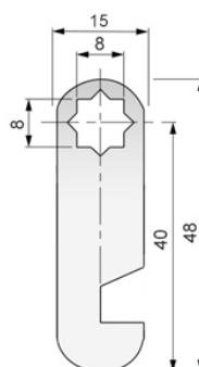
Rygiel hakowy / Hook cam plate
