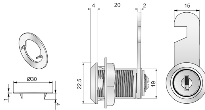
Elementy składowe / Lock Parts
