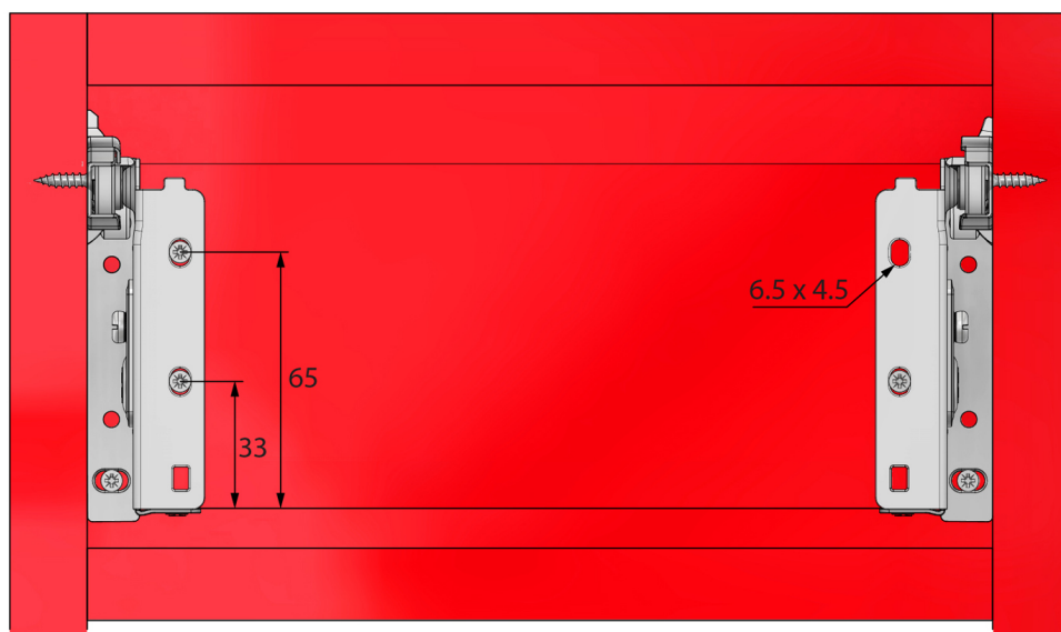
Wymiary montażowe tylnego łącznika / Rear mounting dimensions
