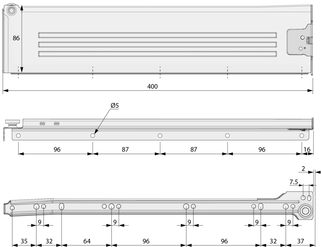
Wymiary montażowe przedniego łącznika / Front mounting dimensions
