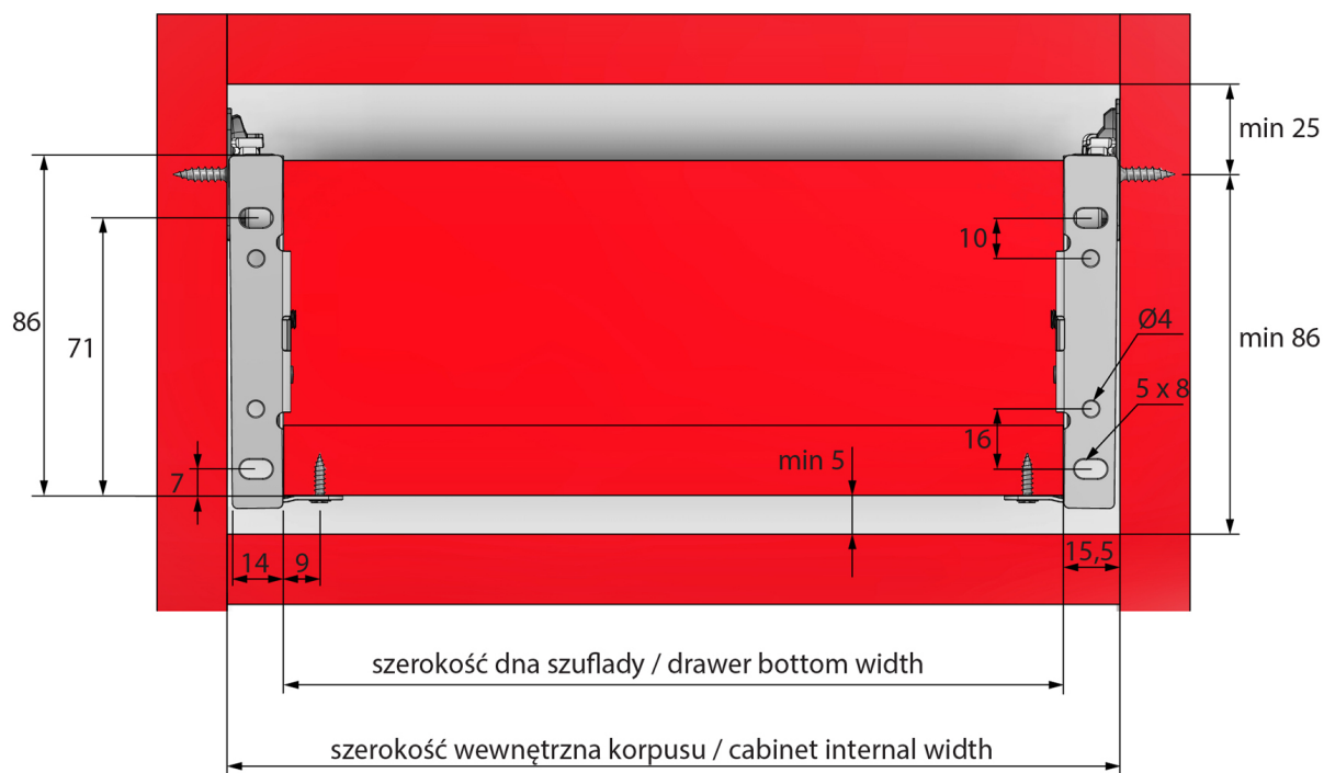
Wymiary montażowe przedniego łącznika / Front mounting dimensions
