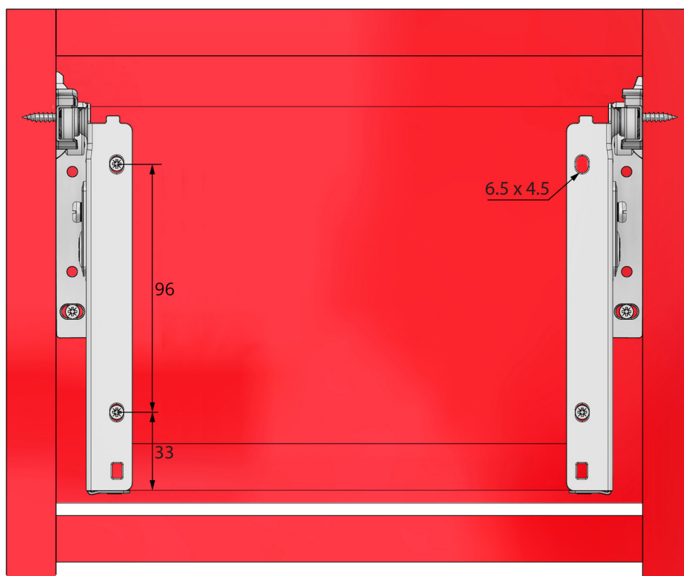
Wymiary montażowe tylnego łącznika / Rear mounting dimensions
