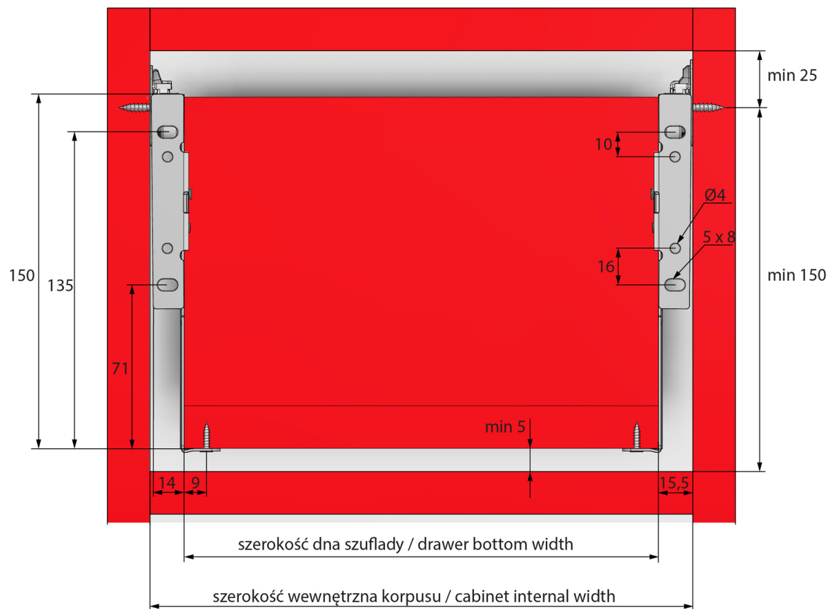
Wymiary montażowe przedniego łącznika / Front mounting dimensions
