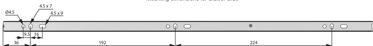
Wymiary montażowe prowadnicy szuflady Mounting dimensions for drawer slide
