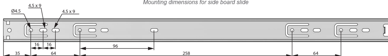
Wymiary montażowe prowadnicy korpusu Mounting dimensions for side board slide
