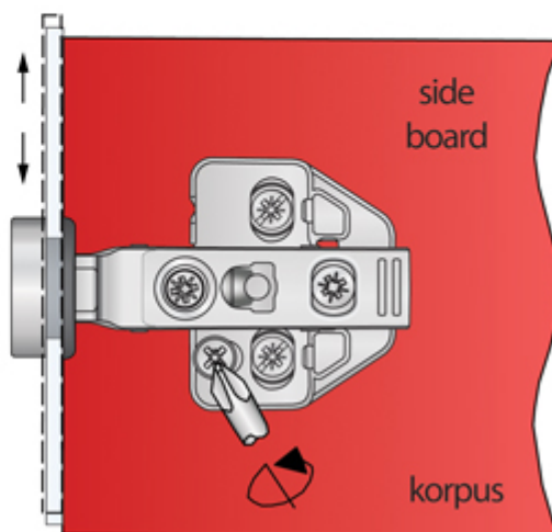
Regulacja wysokości / Height adjustment
