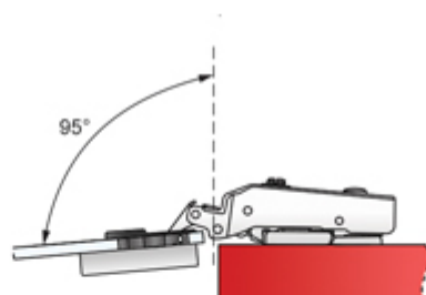
drzwi otwarte / door opened
