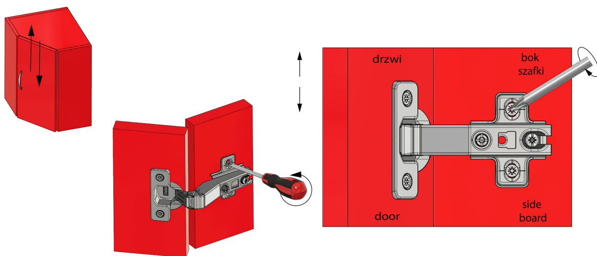
Regulacja wysokości / Height adjustment
