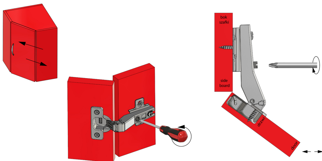
Regulacja boczna / Side adjustment
