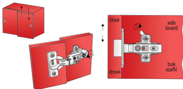
Regulacja wysokości / Height Adjustment
