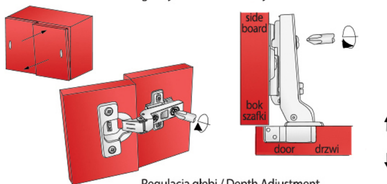
Regulacja głębi / Depth Adjustment
