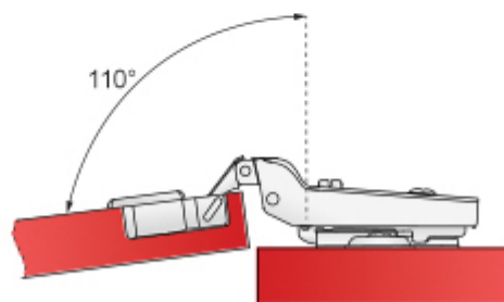
drzwi otwarte / door opened
