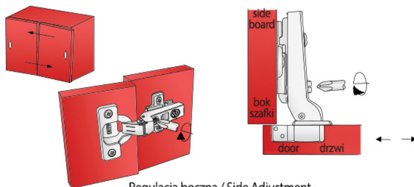
Regulacja boczna / Side Adjustment
