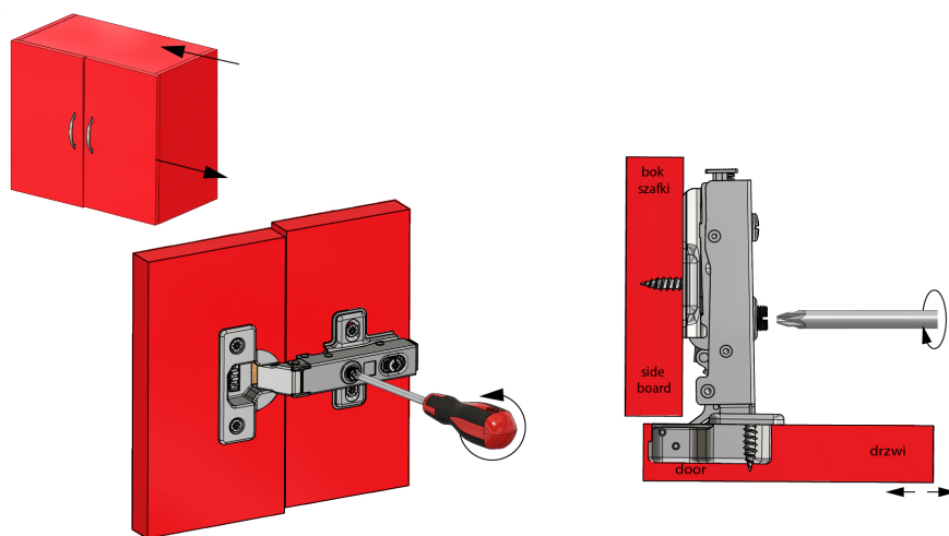
Regulacja boczna / Side adjustment
