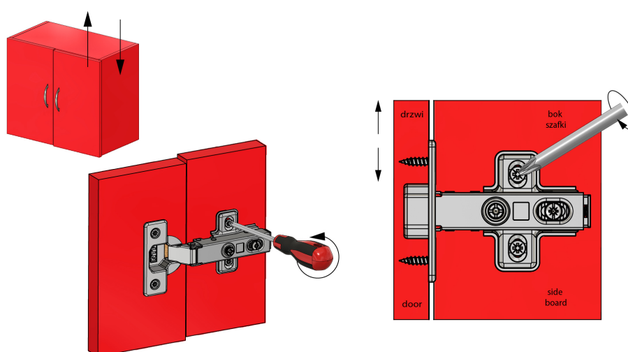
Regulacja wysokości / Height adjustment
