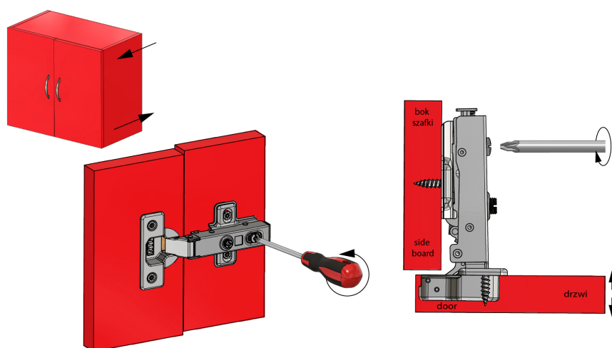
Regulacja głębi / Depth adjustment
