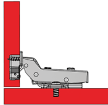
drzwi zamknięte / door close
