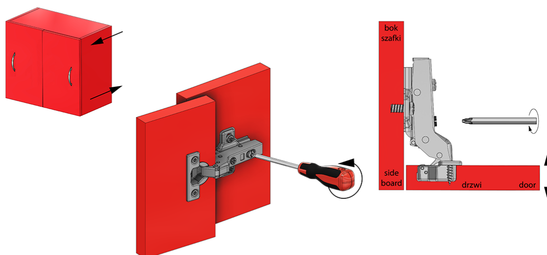
Regulacja głębi / Depth adjustment
